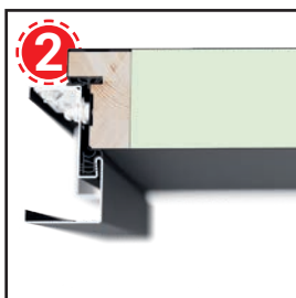
Foaie de ușă din oțel cu ranforsare din lemn și miez din vată minerală
