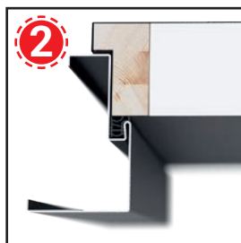
Foaie de ușă din oțel cu ranforsare din lemn și miez din polistiren
